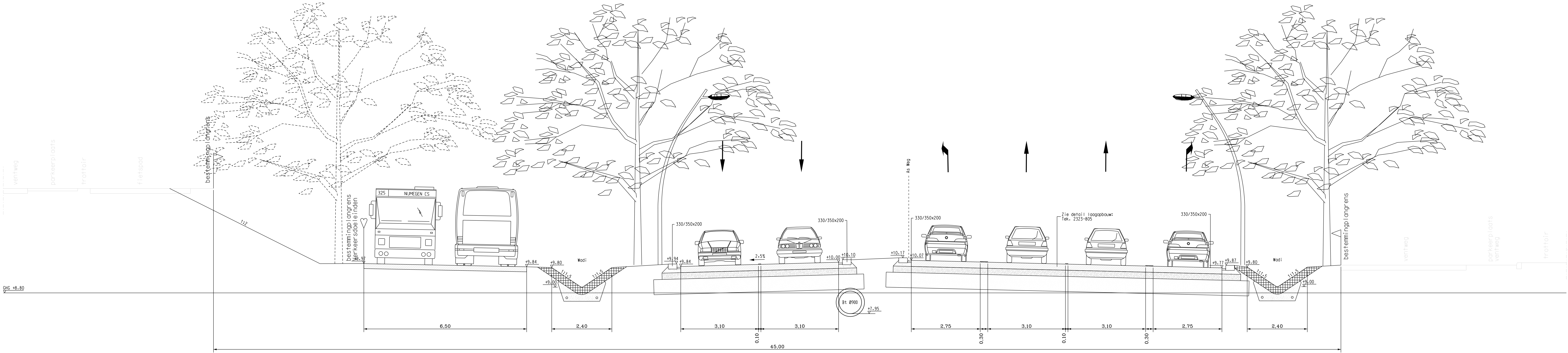
Dwarsprofiel 3-3 Schaal 1:50
